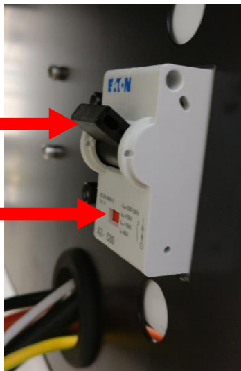
Figura 58 – Sollevare la leva dell'interruttore QB1
