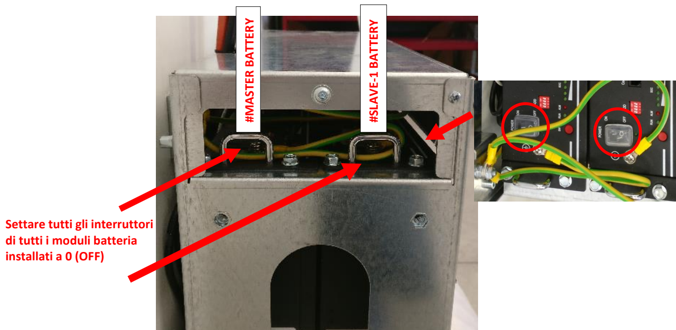
Figura 87 – Posizionare su "0" tutti gli interruttori di tutti i moduli batteria installati sul sistema di accumulo
