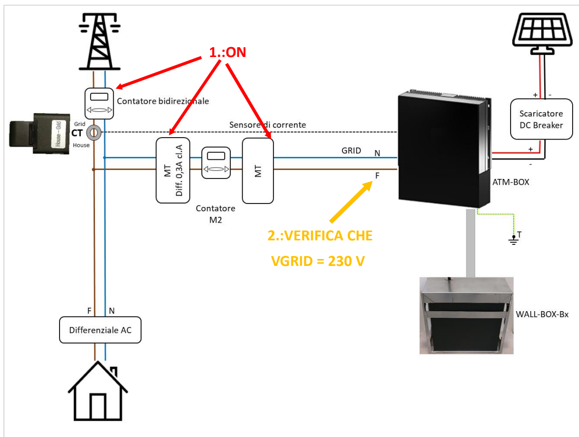
Figura 55 – Preparazione all'attivazione del sistema di accumulo; ripristinare le protezioni elettriche disattivate
