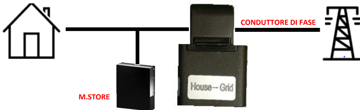
Figura 41 - CT: rispettare il verso di installazione
