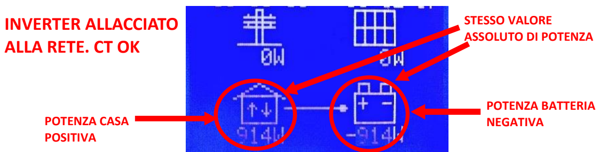
Figura 65 – Visualizzazione corretta con inverter allacciato alla rete
