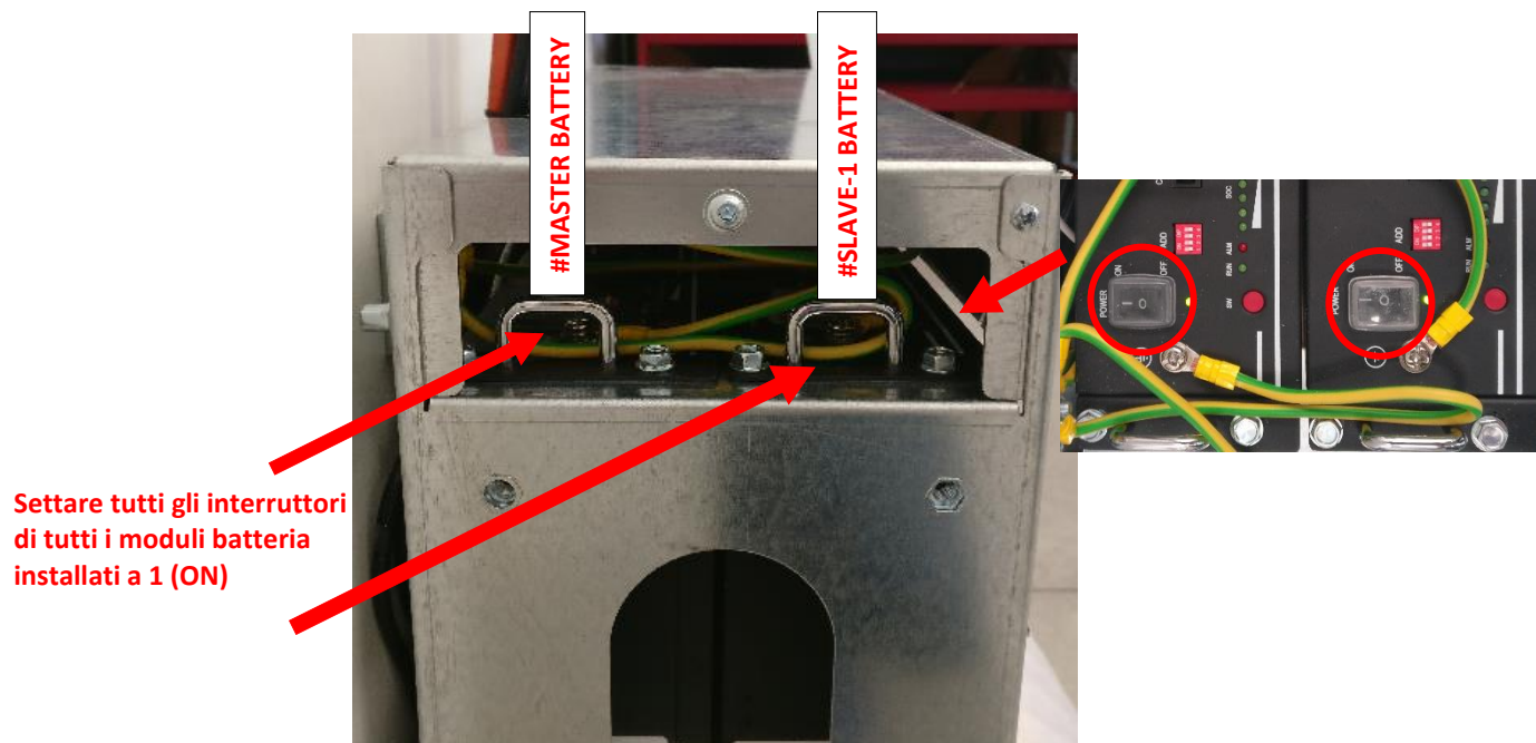
Figura 56 – Posizionare su “1” tutti gli interruttori di tutti i moduli batteria installati sul sistema di accumulo
