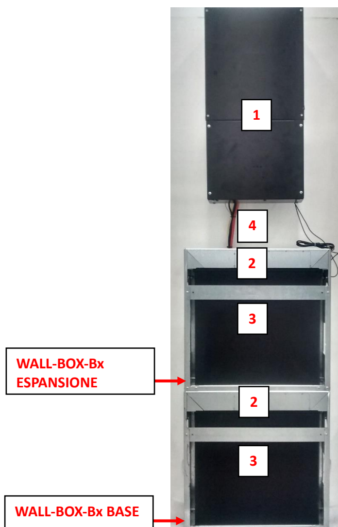
Figura 1 – Composizione sistema
