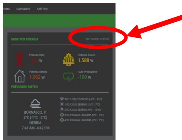
Figura 82 - Controllo impianto da remoto
