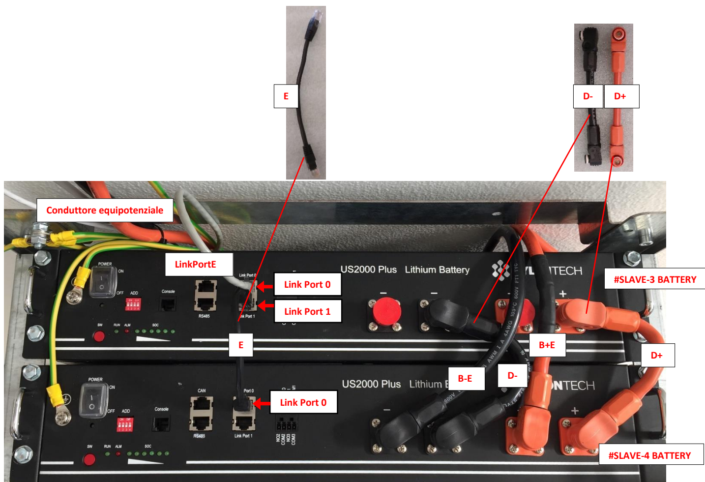
Figura 33 – I collegamenti necessari sul WALL-BOX-Bx ESPANSIONE
