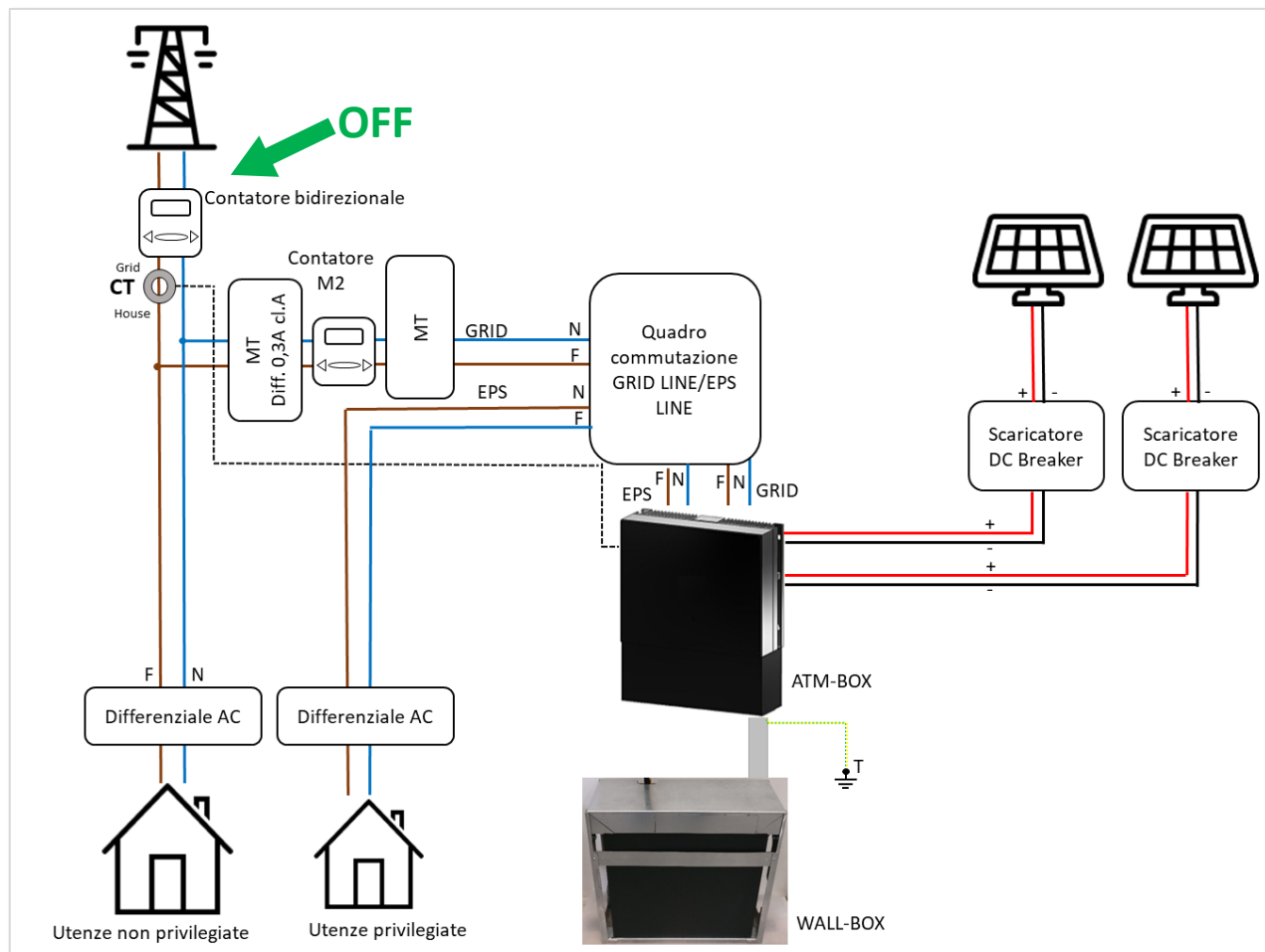
Figura 69 - Simulazione di Black out della rete elettrica nazionale per testare la funzione di EPS dell'accumulatore
