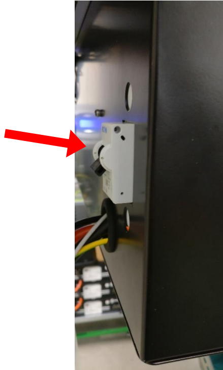
Figura 84 – Abbassare la leva dell'interruttore QB1 per attivare il M.Store
