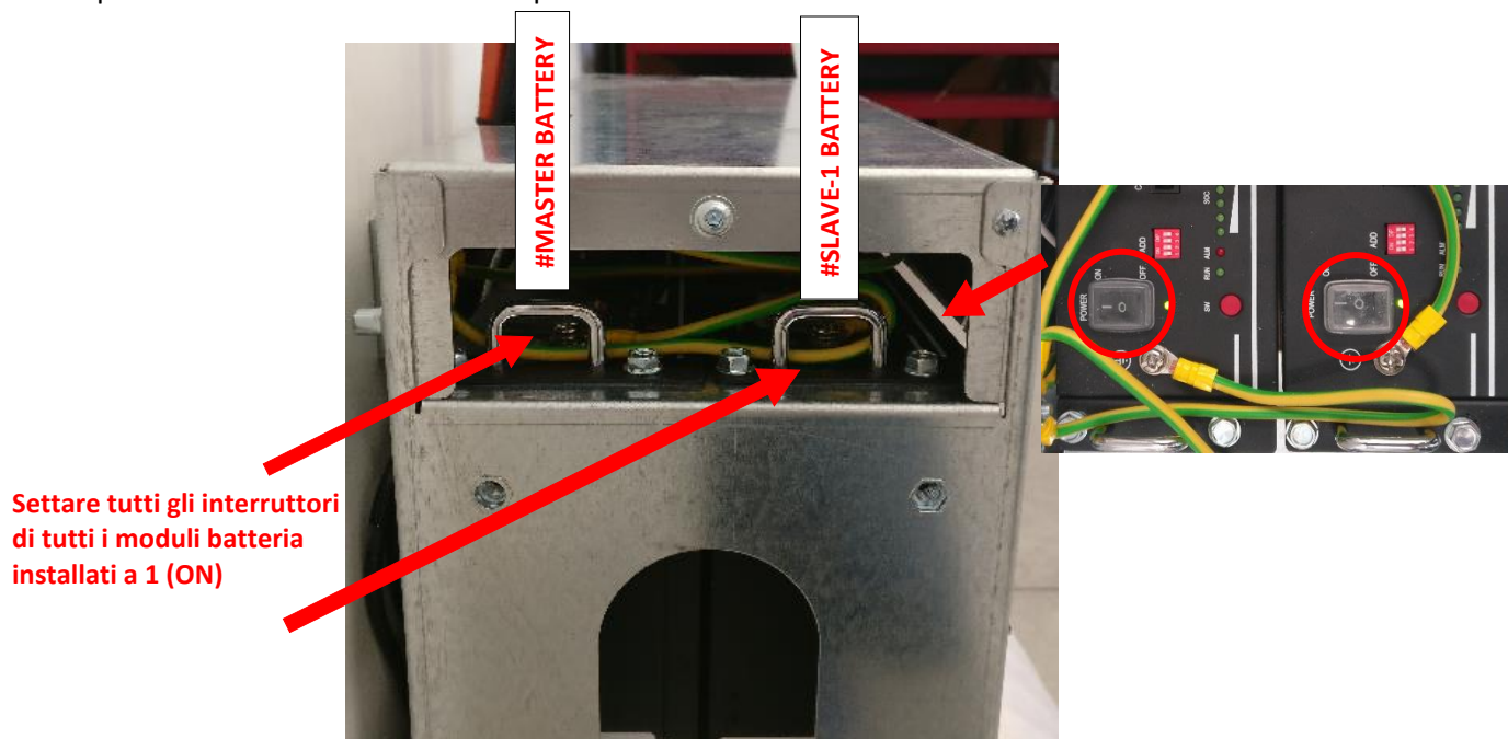
Figura 88 – Posizionare su "1" tutti gli interruttori di tutti i moduli batteria installati sul sistema di accumulo
