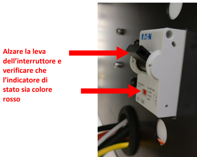
Figura 85 – Sollevare la leva dell'interruttore QB1 per attivare il M.Store
