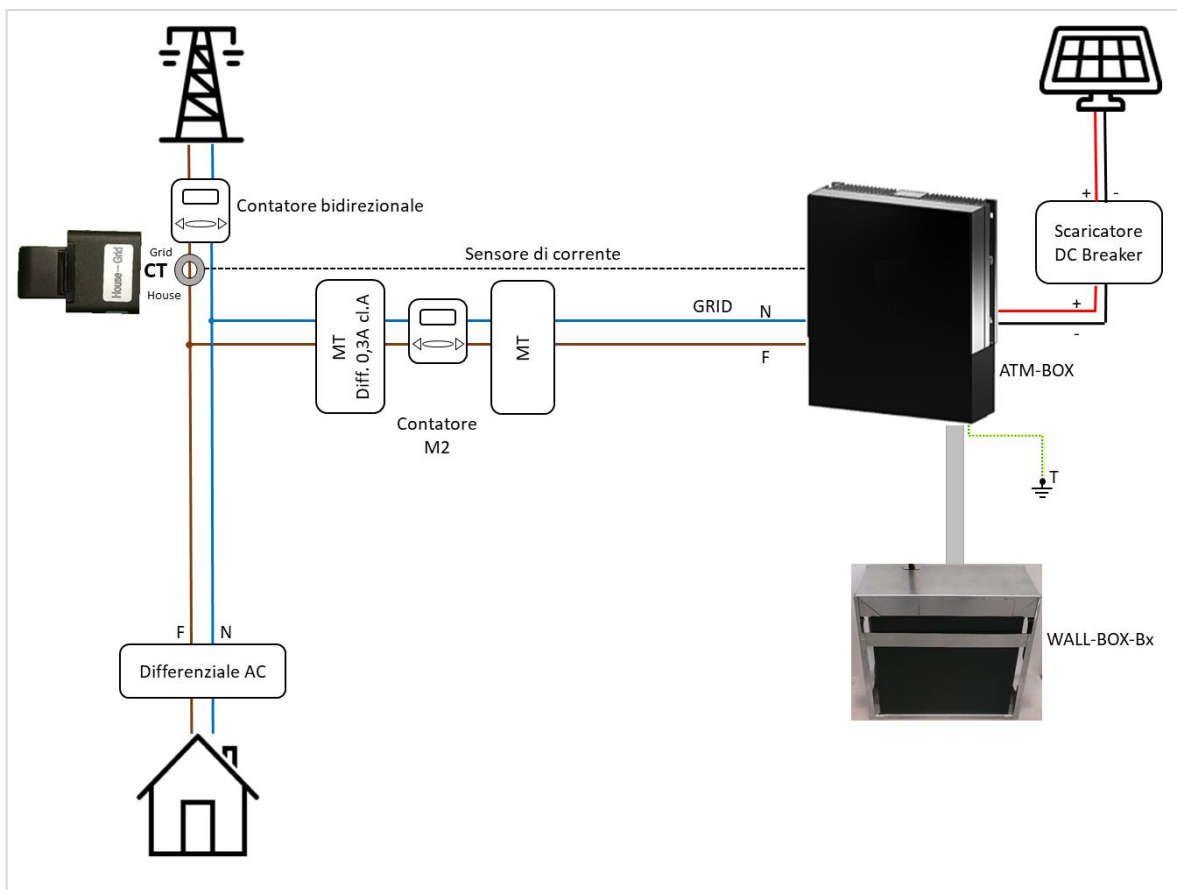
Figura 42 - Sensore CT: rispettare il verso di installazione
