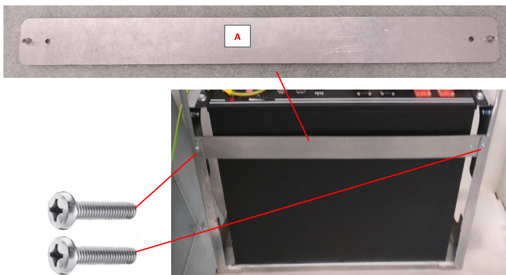
Figura 25 – Installazione staffa segregazione batterie sul WALL-BOX-Bx BASE
