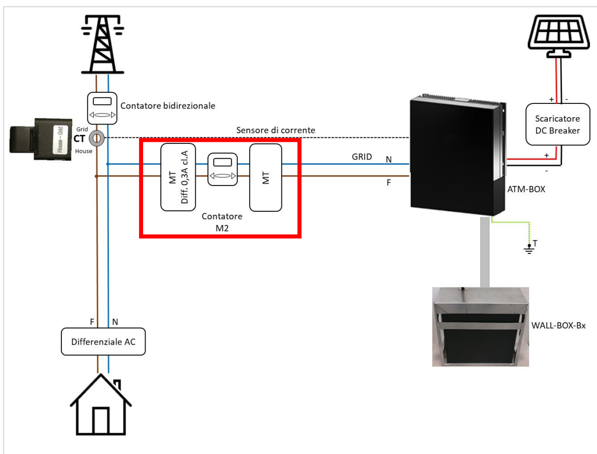
Figura 52 - Quadro elettrico da installare sulla linea “GRID”
