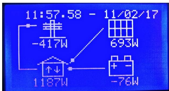
Figura 67 - Visualizzazione prima che venga azzerata la potenza visualizzata sotto l'icona TRALICCIO da parte dell'accumulo
