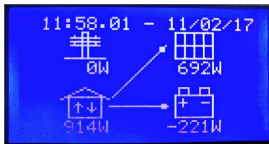
Figura 68 - Visualizzazione dopo che è stata azzerata la potenza visualizzata sotto l'icona TRALICCIO da parte dell'accumulo
