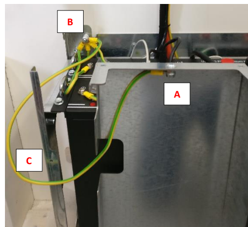
Figura 27 – Collegamento equipotenziale coperchio
