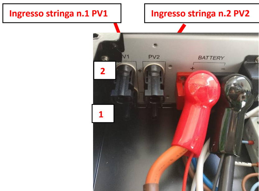
Figura 50 - Collegamento connettori MC4
